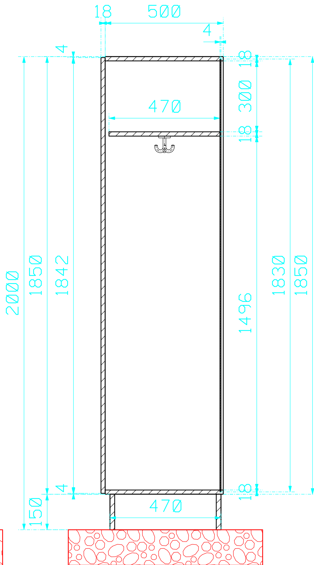
Doorsnede A.-A. D1-garderobekast.
